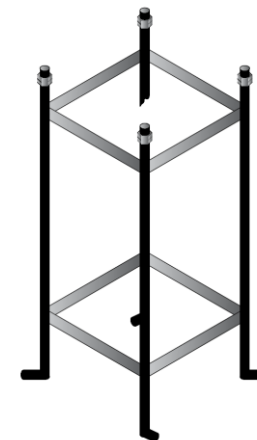
Chumbador para postes flangeados.
